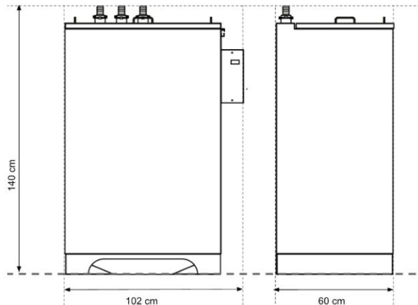
Vorderansicht
