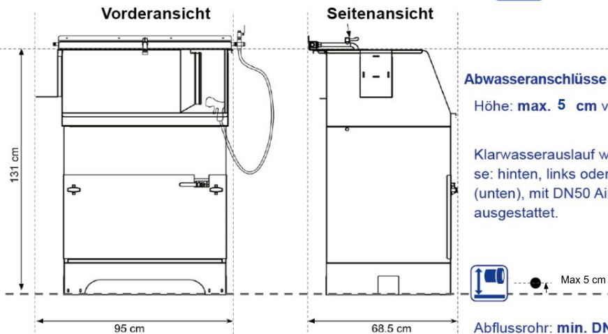
Ansicht mit GS Wasseranschluss Tapsy-1
